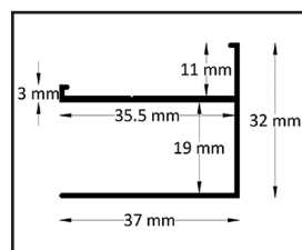
Wandprofil
