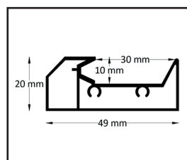
Binäres Profil
