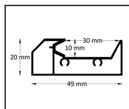
Profil prowadnicy
