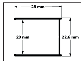
Wandprofil
