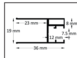
estes Glasprofil
