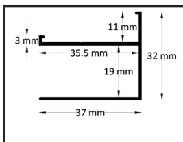
Festes Wandprofil
