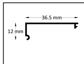
Wandprofilabdeckung
