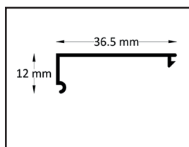
Cubierta perfil muro
