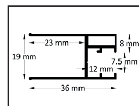
Perfil de cristal fijo
