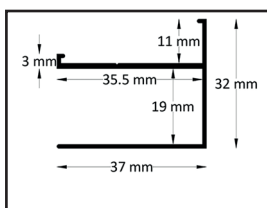
Profilo muro parete fissa
