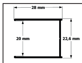
Profilo muro
