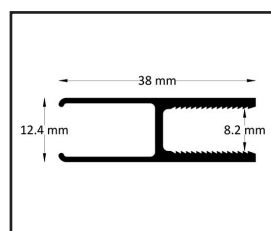
Festseitiges Glasprofil
