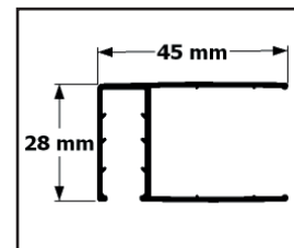
Profil narożny
