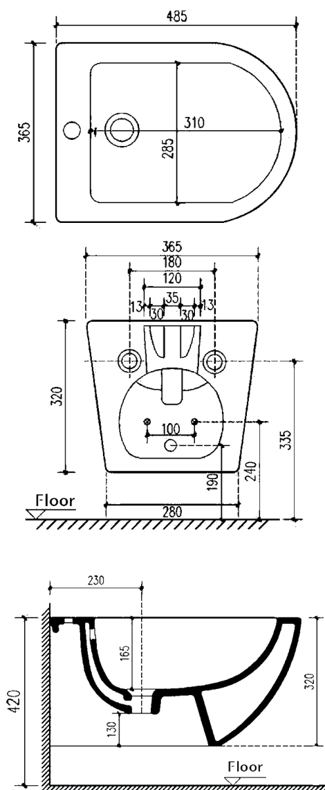
BIDET (art.GIO.33)
