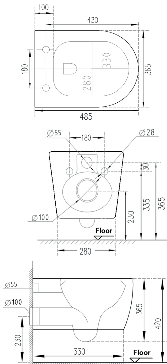
TOILET (art.GIO.32)
