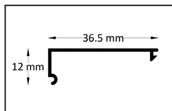
Couverture profilé mural
