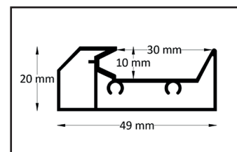
Profil prowadnicy
