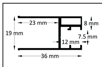
Profil szkła stałego
