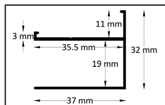
Profil przyścienny
