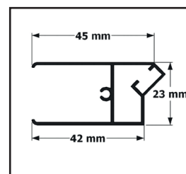
Profilo calamita
