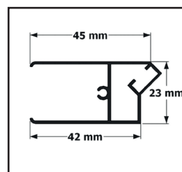
Profil magnetyczny
