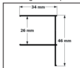
Wandprofil
