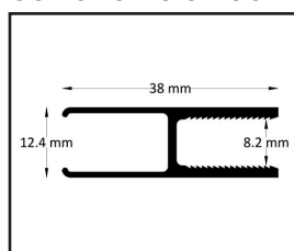
Festseitiges Glasprofil
