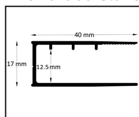
Festseitiges Wandprofil
