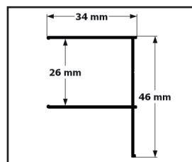
Profil wall
