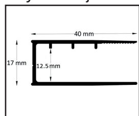
Profil przyścienny szkła stałego
