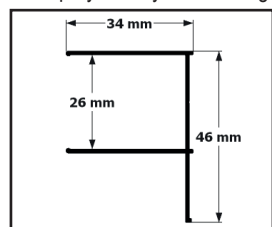
Profil przyścienny
