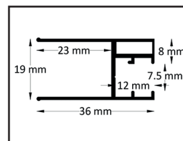
stes Glasprofil
