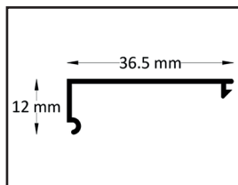
Wandprofilabdeckung
