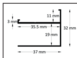
Profilé mural fixe
