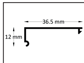
Couverture profilé mural
