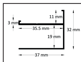
Profilo muro parete fissa
