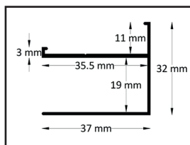
Profil przyścienny ścianka stała
