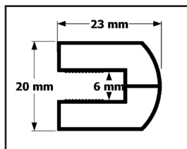
Glasprofil
