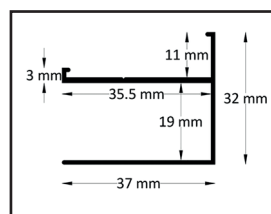
Festes Wandprofil
