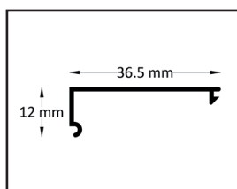
Wandprofilabdeckung
