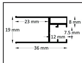
Festes Glasprofil
