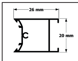
Profil des Scharniers
