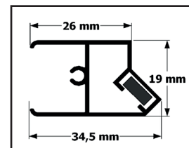
Magnet-Schließprofil
