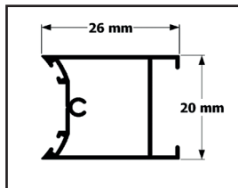
Profilo cerniera
