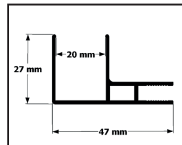
Profilo angolare
