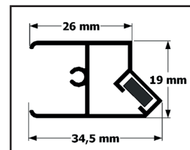
Profil magnesowy zamykający
