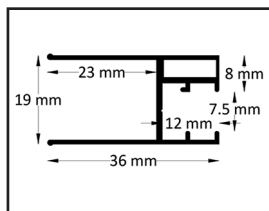
Profil szkła stałego
