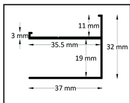
Profil przyścienny ścianki stałej
