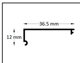
Pokrywa profilu przyściennego
