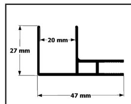
Profil kątowy
