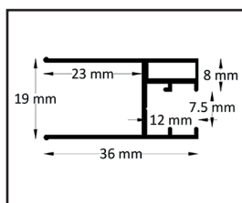
Festes Glasprofil
