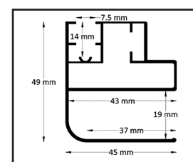
Eckprofil
