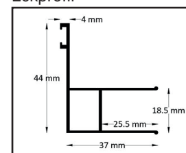
Profil des Türverschlusses
