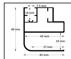
Profilé d'angle
