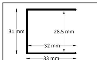
Türseitiges Wandprofil
