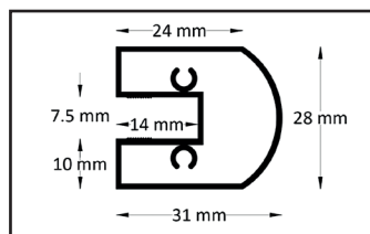
Glas-Drehprofil
