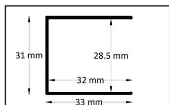
Perfil pared lateral de la puerta
