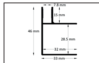
Perfil de esquina
