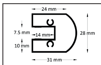
Perfil giratorio de cristal
