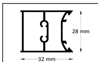
Perfil de bisagra
