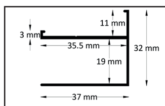
Profil przyścienny ścianka stała
