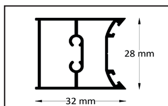
Profil zawiasu
