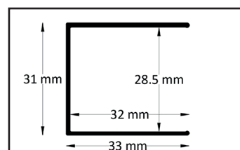
Profil przyścienny strony drzwi
