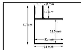
Profil kątowy
