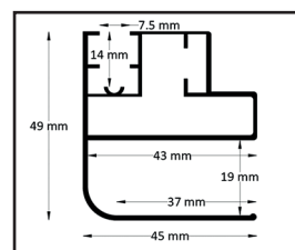
Profilo angolare
