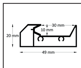
Profilo binario
