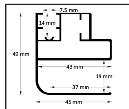
Profil kątowy
