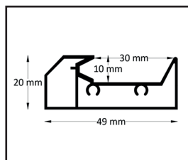
Profil szynowy
