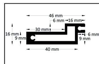
Gleitschiene für Räder
