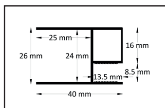
Perfil fijo de estanqueidad del vidrio
