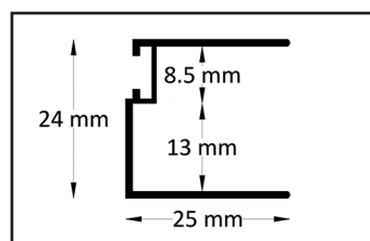
Perfil de pared lateral fijo
