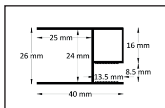
Profilé d'étanchéité en verre fixe
