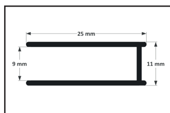
Profil de fermeture de porte
