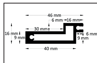
Schienenstange der Rollen
