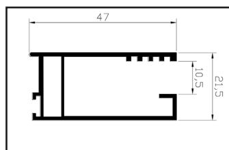
Perfil de pared lado fijo
