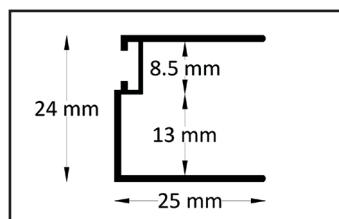
Profil przyścienny po stronie drzwi
