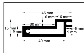
Szyna prowadząca z rołkami
