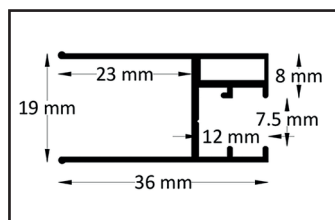
Festes Glasprofil
