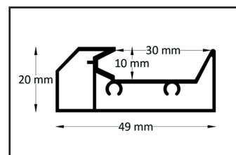
Binäres Profil
