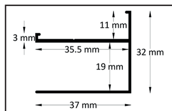
Wandprofil
