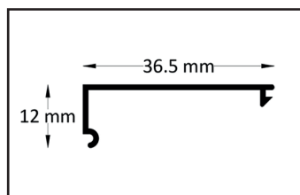
Wandprofilabdeckung
