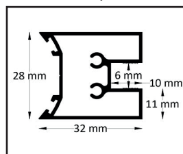
Festes Wandprofil
