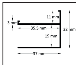
Festes Wandprofil
