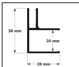
Eckprofil
