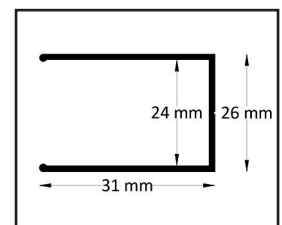
Festes Glaswandprofil
