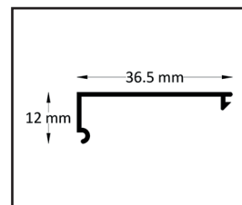
Wandprofilabdeckung
