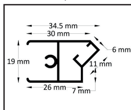
Perfil del percutor magnético
