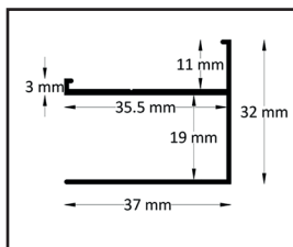
Perfil mural fijo
