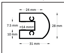
Perfil de cristal giratorio
