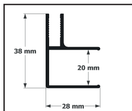
Profilo angolare
