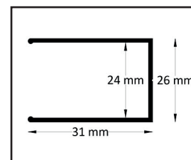
Profilo muro vetro fisso
