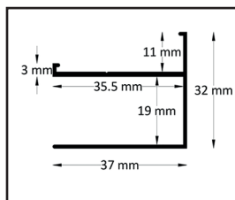
Profilo muro parete fissa
