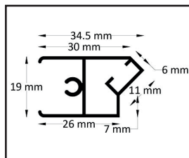
Profil magnetyczny zamykający
