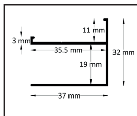
Profil przyścienny ścianki stałej
