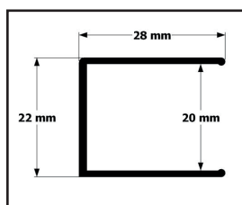
Türseitiges Wandprofil
