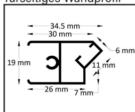
Profil des Magnetstürmers
