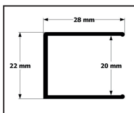
Perfil pared lateral de la puerta
