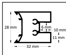
Profil de la charnière
