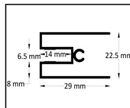
Profilo vetro fisso
