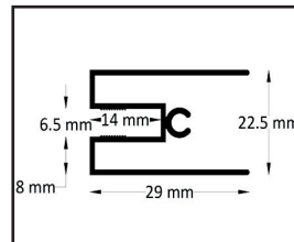
Profil szkła stałego
