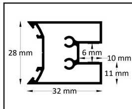
Profil zawiasu
