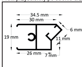
Profil magnetyczny zamykający
