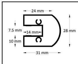
Profil szkła obrotowego
