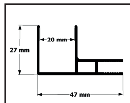
Eckprofil
