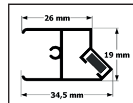
Perfil del percutor magnético
