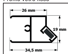
Profilo riscontro calamita
