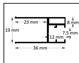
Profilo vetro fisso
