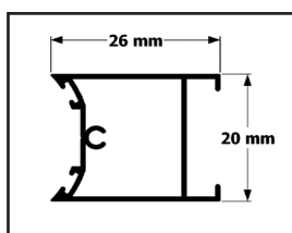
Profilo
