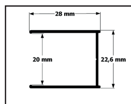
Profilo muro
