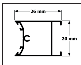
Profil za
