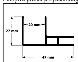
Pokrywa profilu przyściennego
