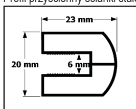
Profil przyścienny ścianki stałej
